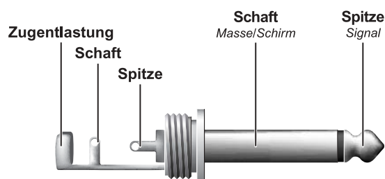
Abb. 4.3: 6,3-mm-Monoklinke
