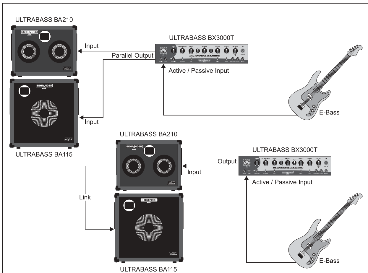
Abb. 3.2: Erweitertes Mono-Setup mit verschiedenen Anschlussoptionen für Lautsprecher
