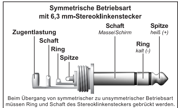
Abb. 4.4: 6,3-mm-Stereoklinkenstecker
