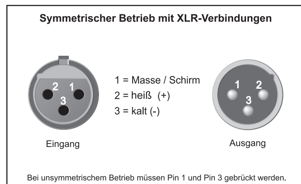
Abb. 4.2: XLR-Verbindungen
