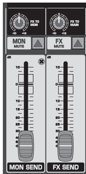
Abb. 2.6: Die Aux Send-Regler der Main-Sektion
