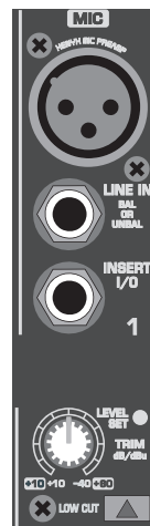
Abb. 2.1: Anschlüsse und Regler der Mic-/Line-Eingänge
