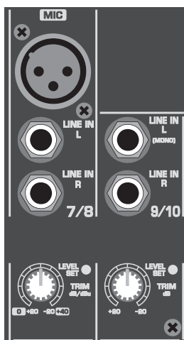
Abb. 2.5: Die Stereokanaleingänge
