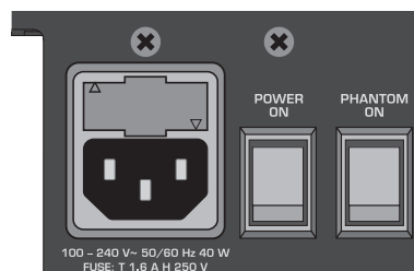
Abb. 2.16: Spannungsversorgung und Sicherung
