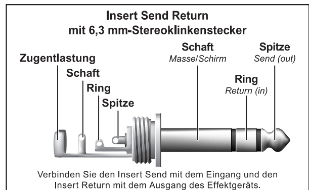
Abb. 4.5: Insert-Send-Return-Stereoklinkenstecker
