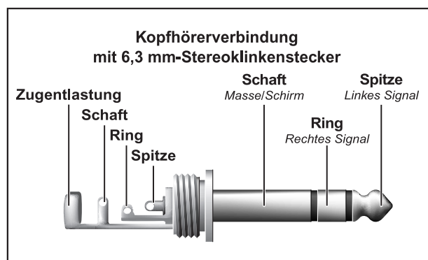
Abb. 4.6: Kopfhörer-Stereoklinkenstecker
