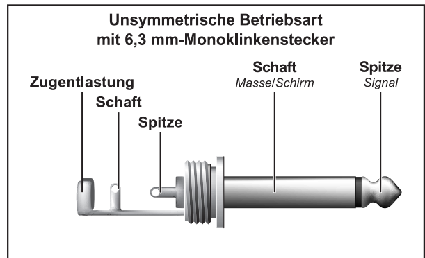
Abb. 4.3: 6,3-mm-Monoklinkenstecker
