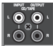
Abb. 2.10: Die 2-Track-Anschlussbuchsen
