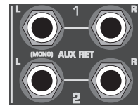
Abb. 2.8: Die Aux Return-Buchsen
