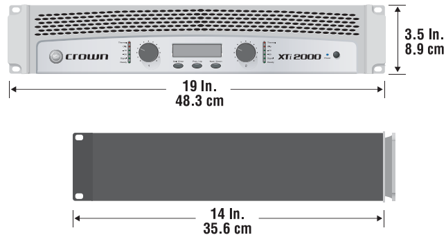
Abb. 2.1 Abmessungen
