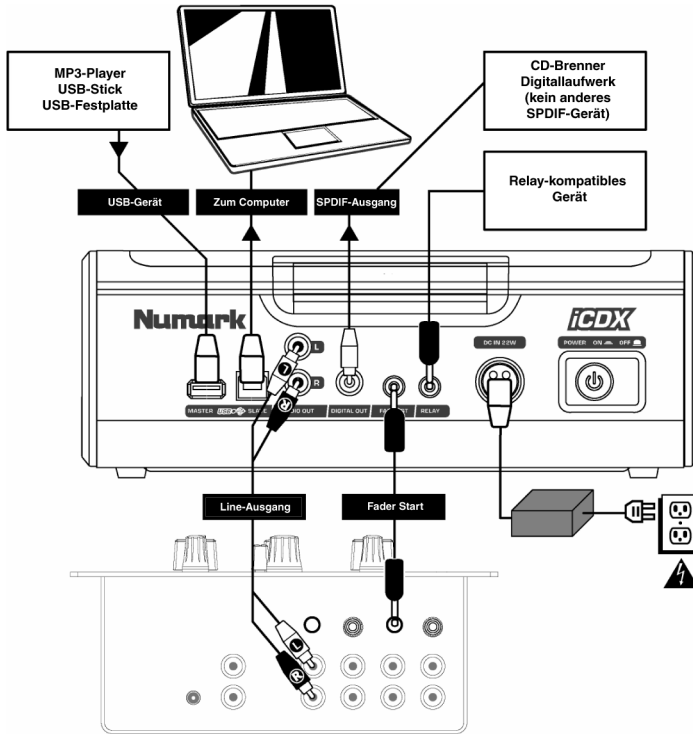
Rückseite des Mixers (MIXER NICHT IM LIEFERUMFANG)
