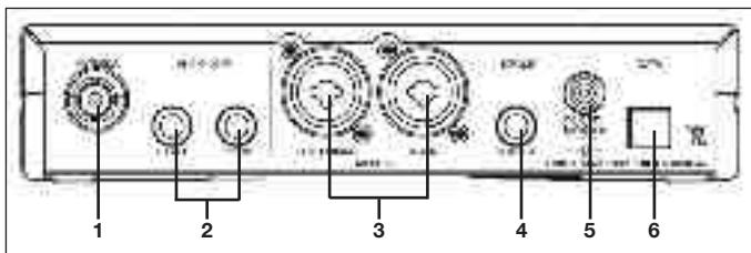
Fig. 3 : Entrées et sorties au dos de l'émetteur
