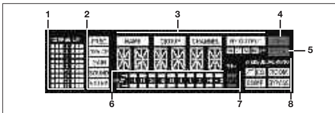
Fig. 2 : Ecran sur le panneau avant de l'émetteur
