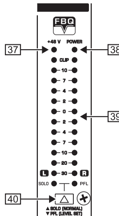
Fig. 2.16: Level meter
