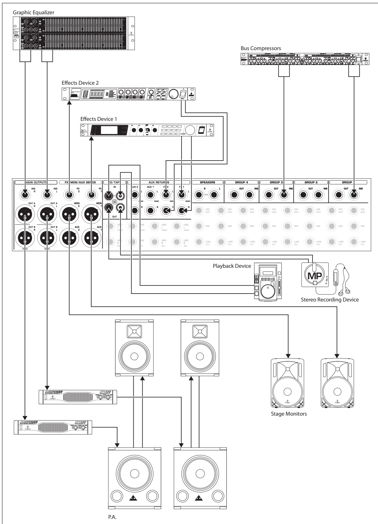
Fig. 2.2: Output wiring
