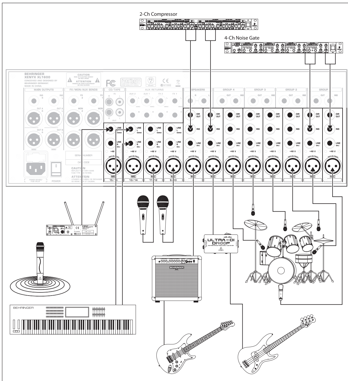
Fig. 2.1: Input wiring
