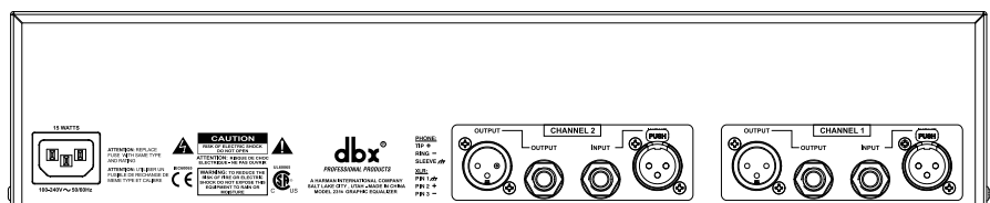
231s - Zweikanaliger grafischer 31-Band-EQ
