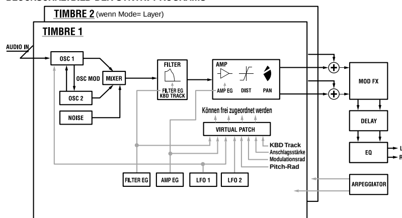
BLOCKSCHALTBILD DER SYNTHI-PROGRAMMS
