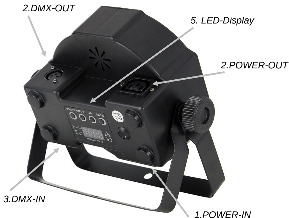
Abb.1 Gehäuserückseite
