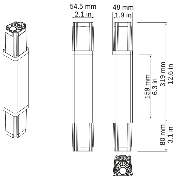
Abbildung 9.2: Abmessungen EVOLVE 50 kurzer Mast
