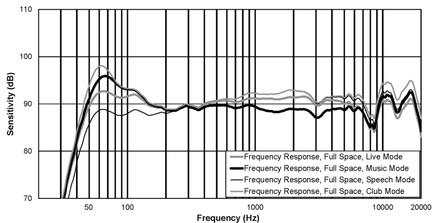
Abbildung 9.3: Frequenzgang EVOLVE 50 (Live, Music, Speech und Club)
