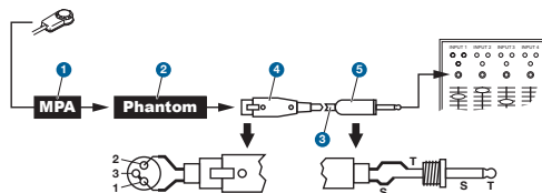
Figura 2: Conexión a entradas no balanceadas
