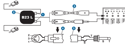
Abbildung 3: Anschluss-Schema mit B23 L
