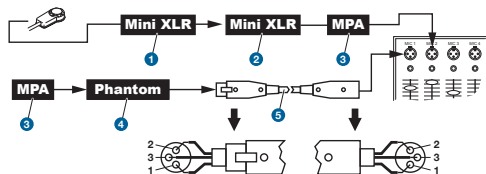
Abbildung 4: Anschluss-Schema mit MPA V L
