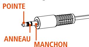
CONNECTEUR MINI JACK 3,5 mm Câblage stéréo
