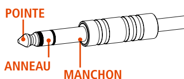
CONNECTEUR JACK TRS 6,35 mm Raccordement mono symétrique
