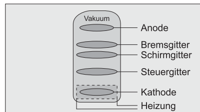
Abb. 4.5: Pentode
