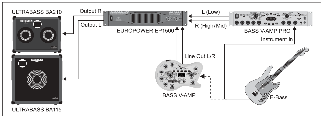
Abb. 3.4: Bi-Amping: Hohe und tiefe Frequenzen werden über die Bassboxen getrennt wiedergegeben
