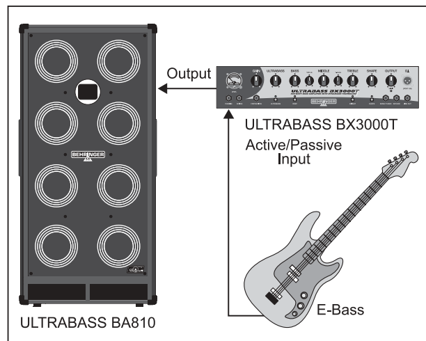
Abb. 3.3: Setup mit der BA810 und dem BX3000T
