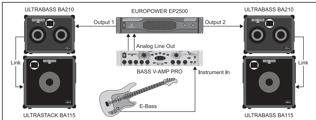
Abb. 3.5: Erweiterte Stereo-Konfiguration
