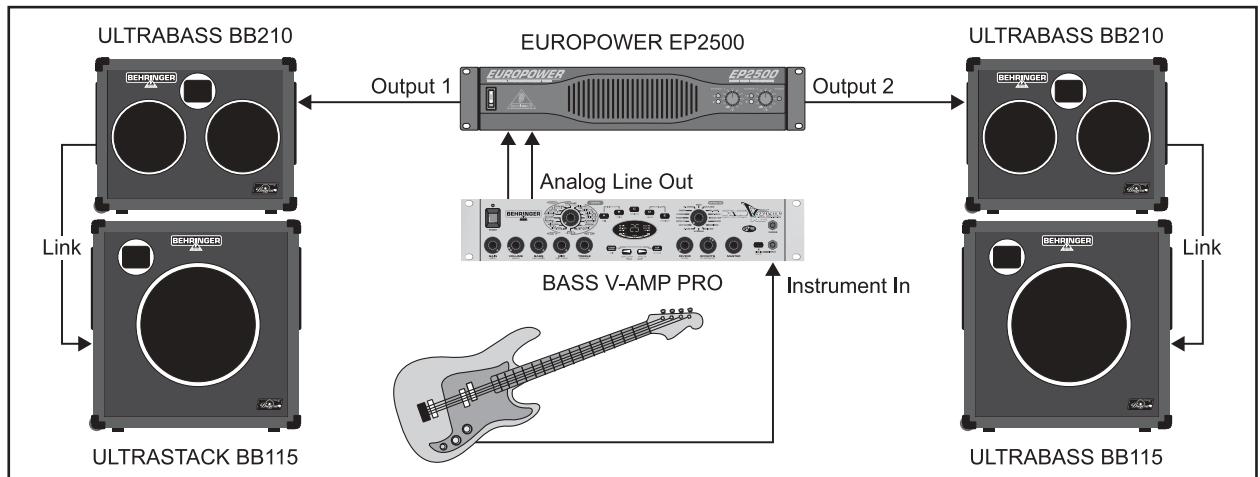
Abb. 3.4: Erweiterte Stereo-Konfiguration
