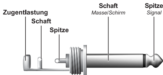
Abb. 8.2: 6,3 mm-Monoklinkenstecker
