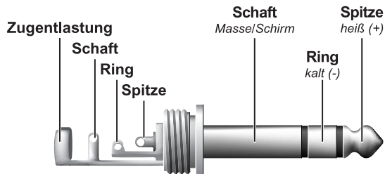
Abb. 8.3: 6,3 mm-Stereoklinkenstecker
