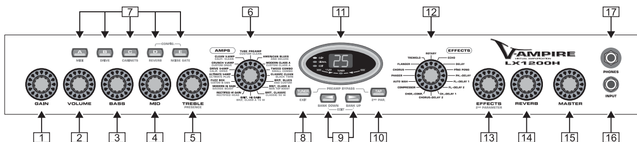
Abb 2.1: Bedienungselemente des V-AMPIRE (Frontseite)
