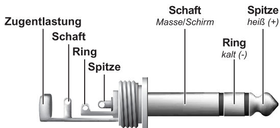
Abb. 8.3: 6,3-mm-Stereoklinkenstecker
