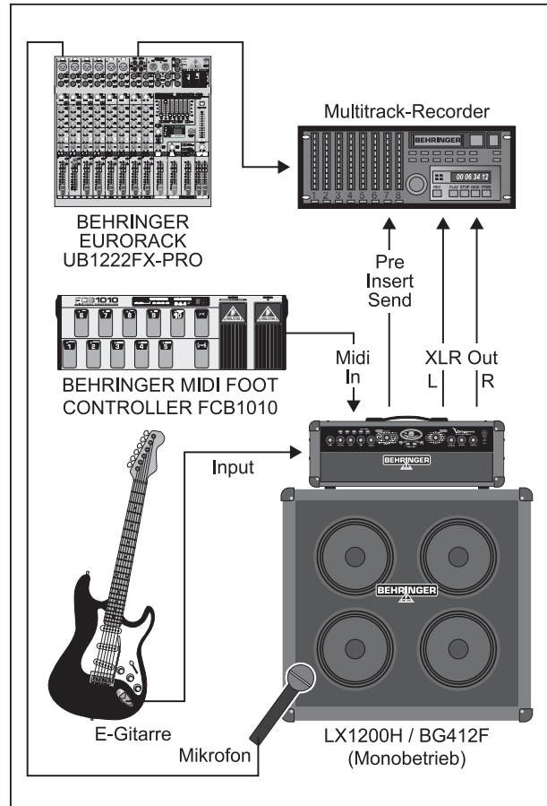
Abb. 3.4: Erweitertes Recording Setup mit Multitrack-Rekorder und Mischpult
