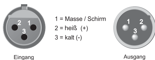
Abb. 8.1: XLR-Verbindungen
