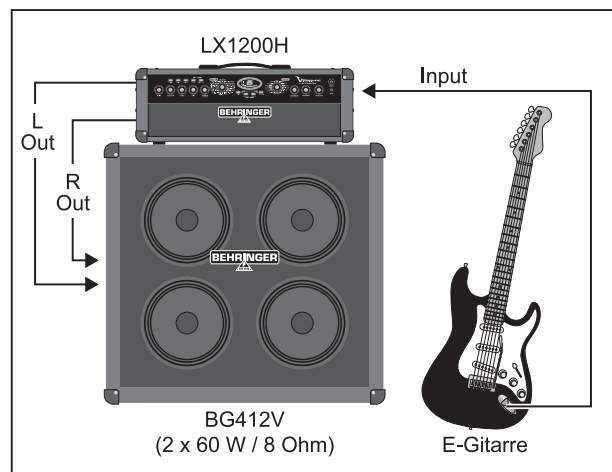
Abb. 3.2: Stereobetrieb an 2 x 8 \Omega Impedanz
