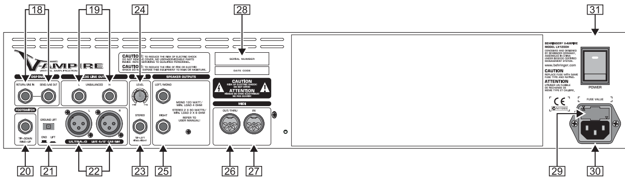
Abb. 2.3: Bedienungselemente des V-AMPIRE (Rückseite)
