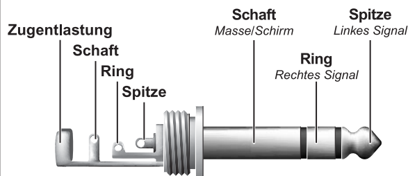
Abb. 8.4: Kopfhörer-Stereoklinkenstecker
