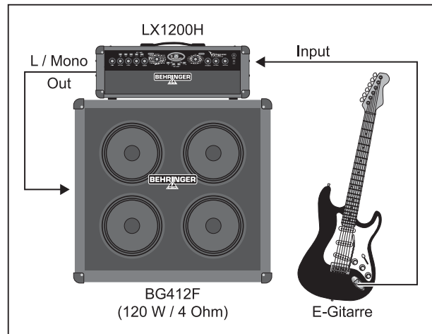
Abb. 3.1: Monobetrieb an 4 \Omega Impedanz
