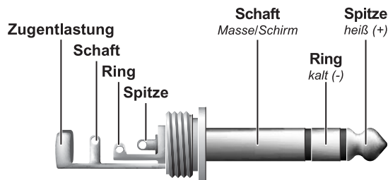
Abb. 8.3: 6,3 mm-Stereoklinkenstecker
