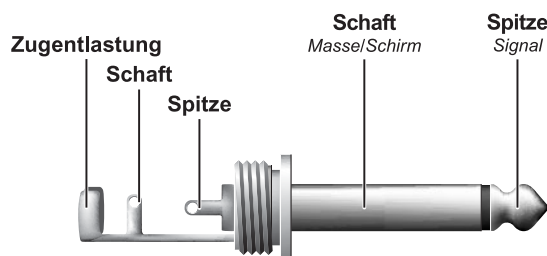
Abb. 8.2: 6,3 mm-Monoklinkenstecker
