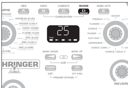
Abb. 4.1: Aufrufen von Presets beim V-AMP 2 (V-AMPIRE und V-AMP PRO ähnlich)
