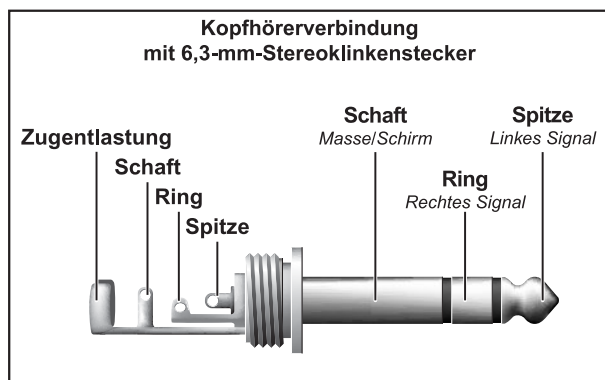
Abb. 8.4: Kopfhörer-Stereoklinkenstecker
