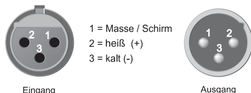
Abb. 8.1: XLR-Verbindungen
