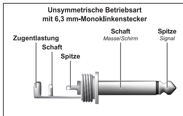
Abb. 6.1: 6,3 mm-Monoklinkenstecker
