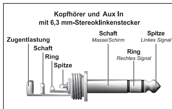
Abb. 6.2: 6,3 mm-Stereoklinkenstecker für AUX und PHONES
