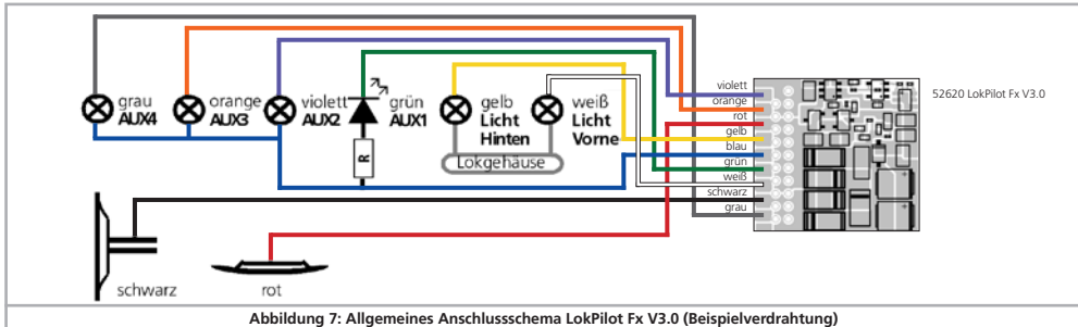
Abbildung 7: Allgemeines Anschlussschema LokPilot Fx V3.0 (Beispielverdrahtung)
