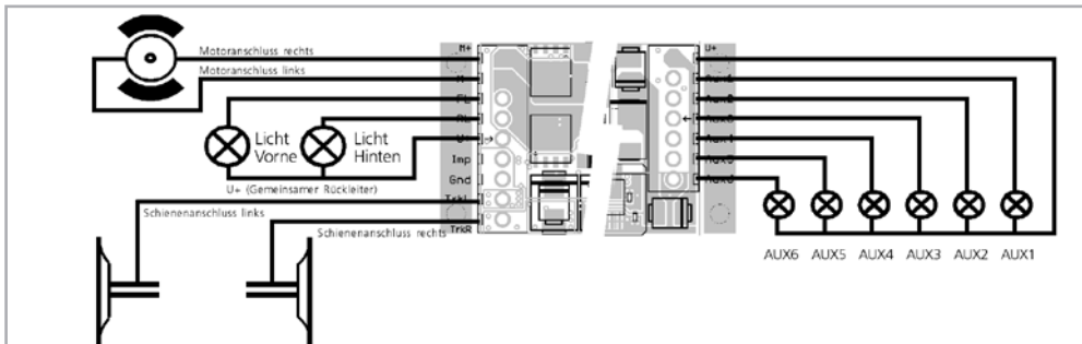
Abbildung 6: Allgemeines Anschlussschema LokPilot XL V3.0 (Beispielverdrahtung)
