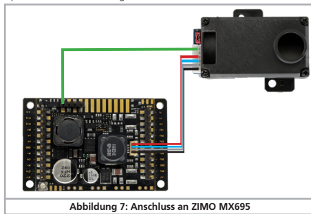
Abbildung 7: Anschluss an ZIMO MX695
