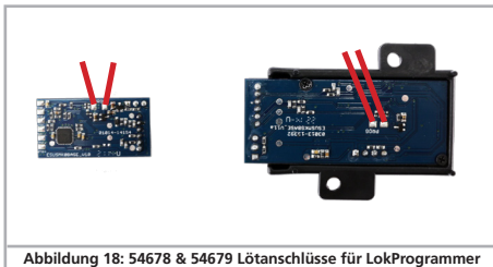
Abbildung 18: 54678 & 54679 Lötanschlüsse für LokProgrammer
