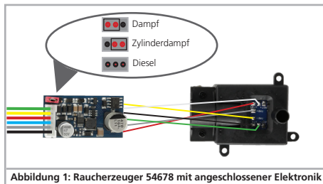
Abbildung 1: Raucherzeuger 54678 mit angeschlossener Elektronik Mittels eines Jumpers kann zwischen der Betriebsart „Diesel“ und „Dampf“ gewechselt werden.
