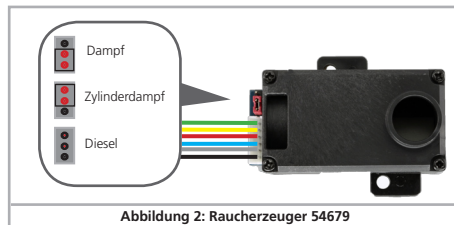
Abbildung 2: Raucherzeuger 54679
