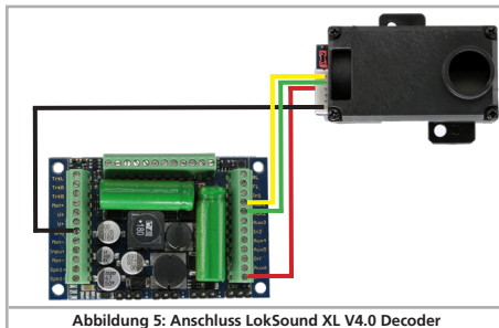
Abbildung 5: Anschluss LokSound XL V4.0 Decoder
