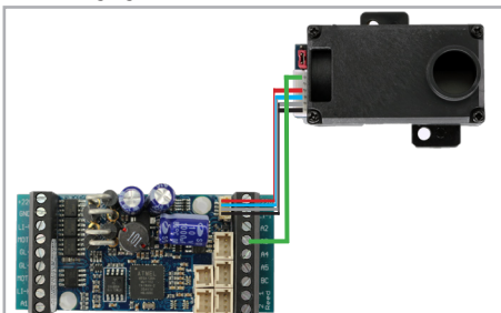
Abbildung 8: Anschluss an Massoth eMotion XLS
