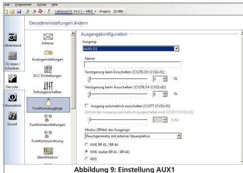
Abbildung 9: Einstellung AUX1
