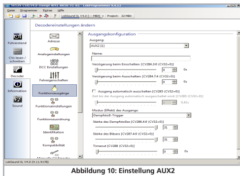
Abbildung 10: Einstellung AUX2
