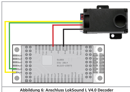
Abbildung 6: Anschluss LokSound L V4.0 Decoder
