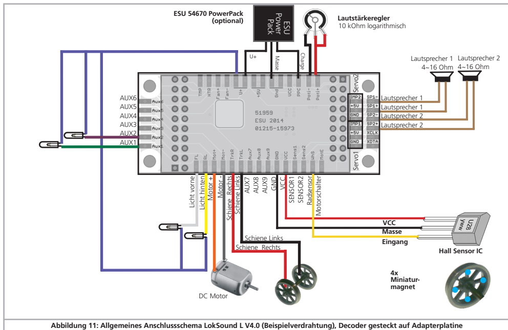
Abbildung 11: Allgemeines Anschlussschema LokSound L V4.0 (Beispielverdrahtung), Decoder gesteckt auf Adapterplatine
