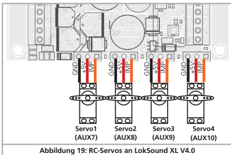
Abbildung 19: RC-Servos an LokSound XL V4.0
