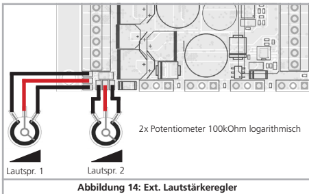
Abbildung 14: Ext. Lautstärkeregler
