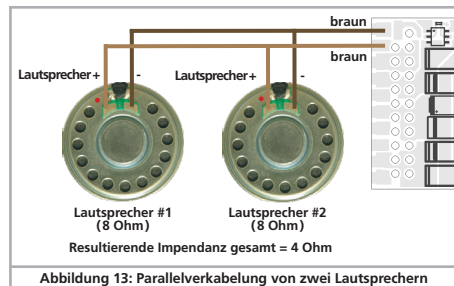
Abbildung 13: Parallelverkabelung von zwei Lautsprechern
