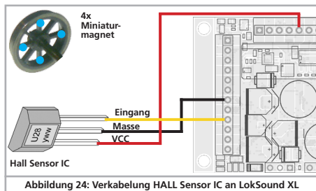
Abbildung 24: Verkabelung HALL Sensor IC an LokSound XL
