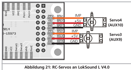
Abbildung 21: RC-Servos an LokSound L V4.0
