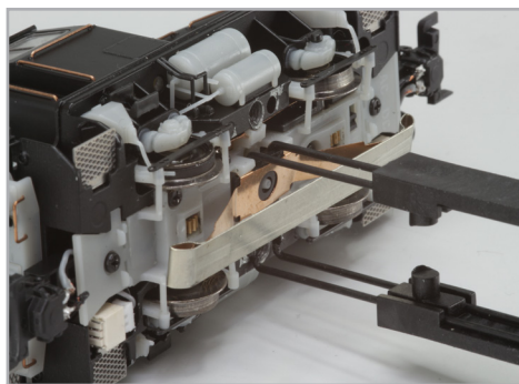
Abbildung 3: Schleifer abziehen
