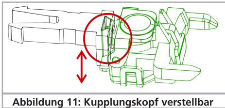
Abbildung 11: Kupplungskopf verstellbar
