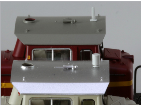
Abbildung 15: Antennen montiert
