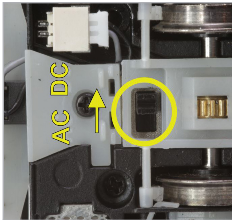
Abbildung 4: Schiebeschalter DC-Betrieb
