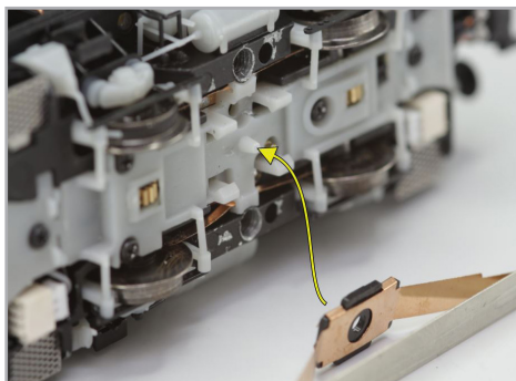
Abbildung 5: Schleifer ansetzen
