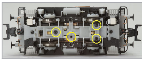
Abbildung 13: Position der Schrauben
