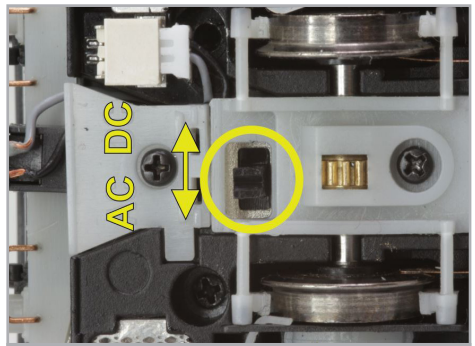
Abbildung 2: Schiebeschalter AC-Betrieb
