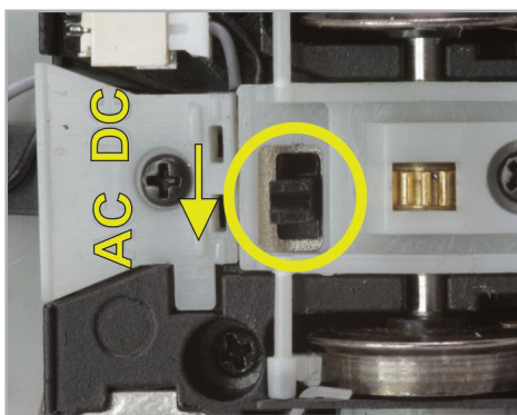
Abbildung 6: Schalter auf AC-Betrieb
