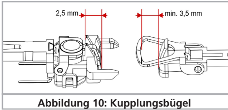
Abbildung 10: Kupplungsbügel
