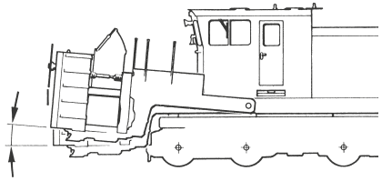
F3 Fräskopf Heben und Senken
