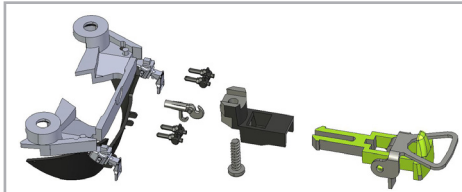
Abbildung 14: Benötigte Teile
