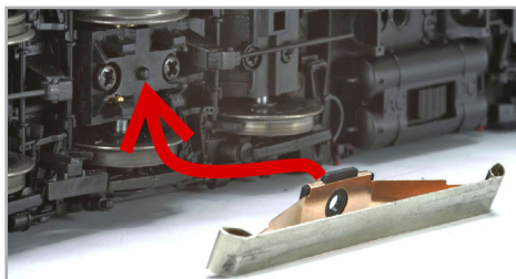
Abbildung 5: Schleifer ansetzen
