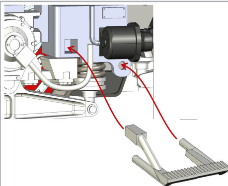
Abbildung 12: Trittstufen montieren
