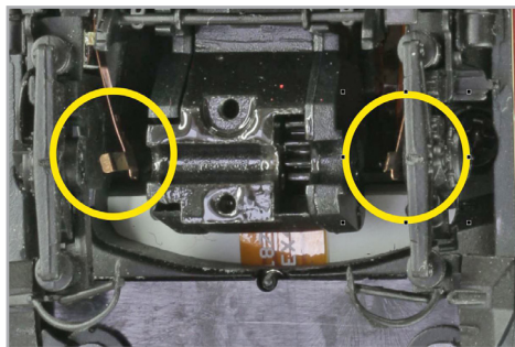
Abbildung 11: Position Radschleifer
