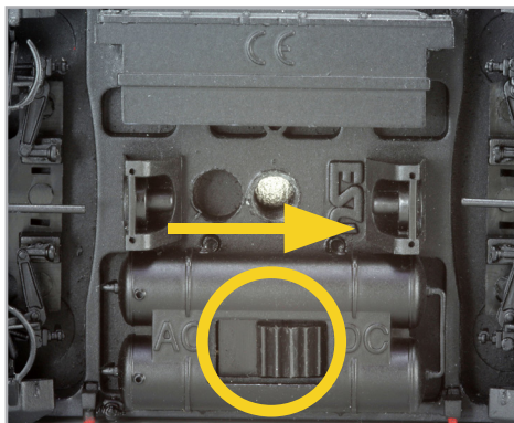
Abbildung 4: Schiebeschalter DC-Betrieb
