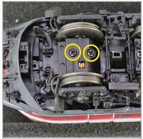
Abbildung 10: Schrauben Getriebedeckel
