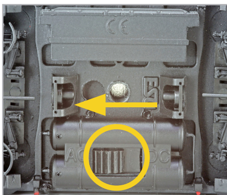
Abbildung 6: Schalter auf AC-Betrieb
