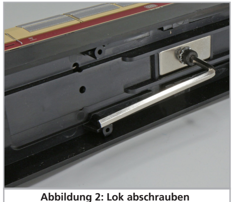
Abbildung 2: Lok abschrauben
